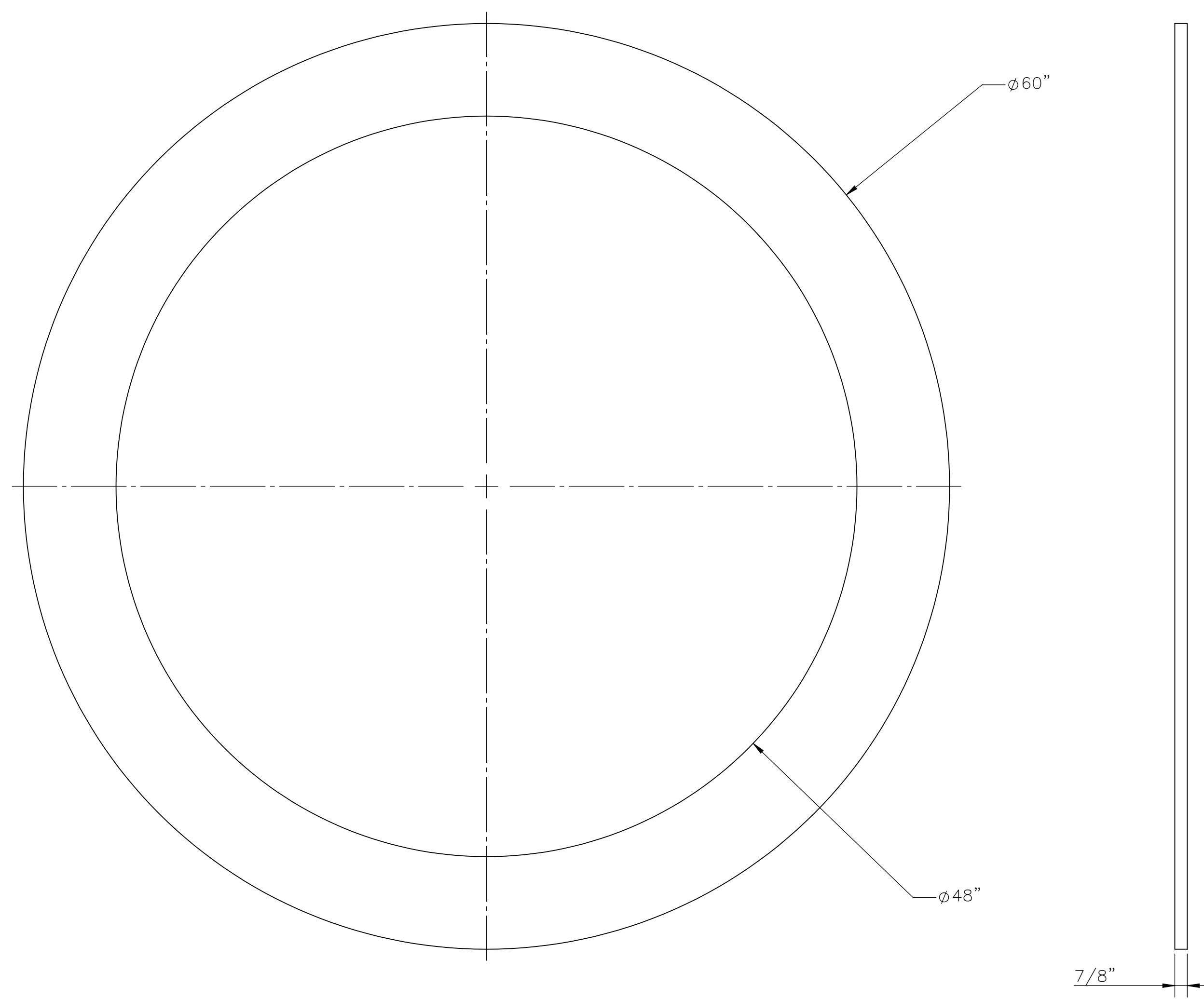
⑤ 48 INCH RISER BOTTOM PLATE SCALE: 2"=1'-0"
