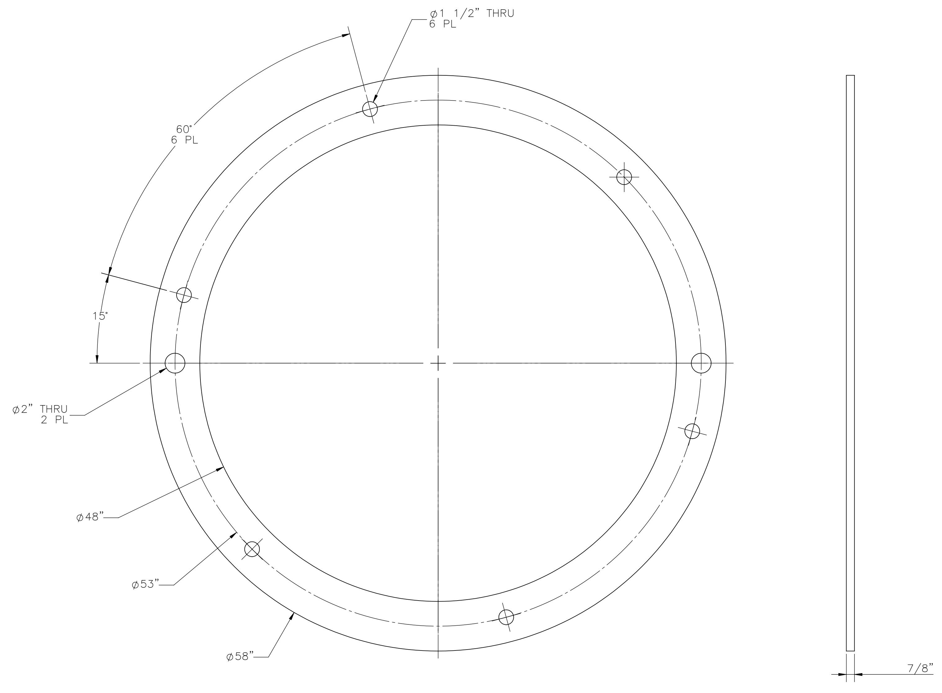
⑥ 48 INCH RISER TOP PLATE SCALE: 2"=1'-0"
