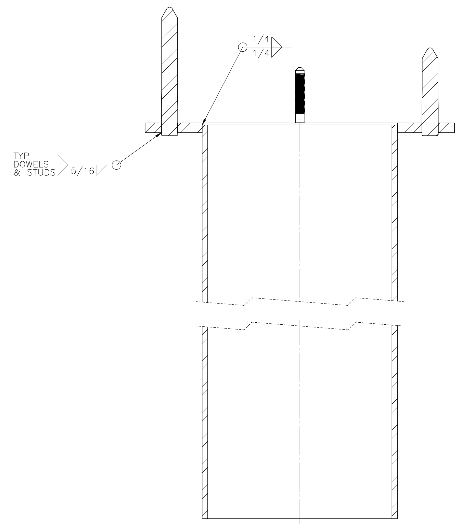
SECTION C-C SCALE: 2"=1'-0"
