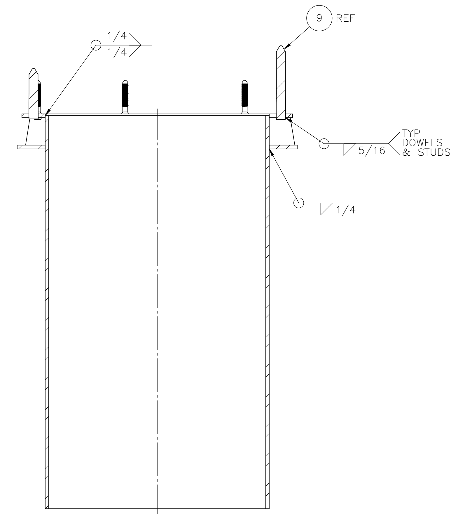
SECTION A-A SCALE: 1"=1'-0"
