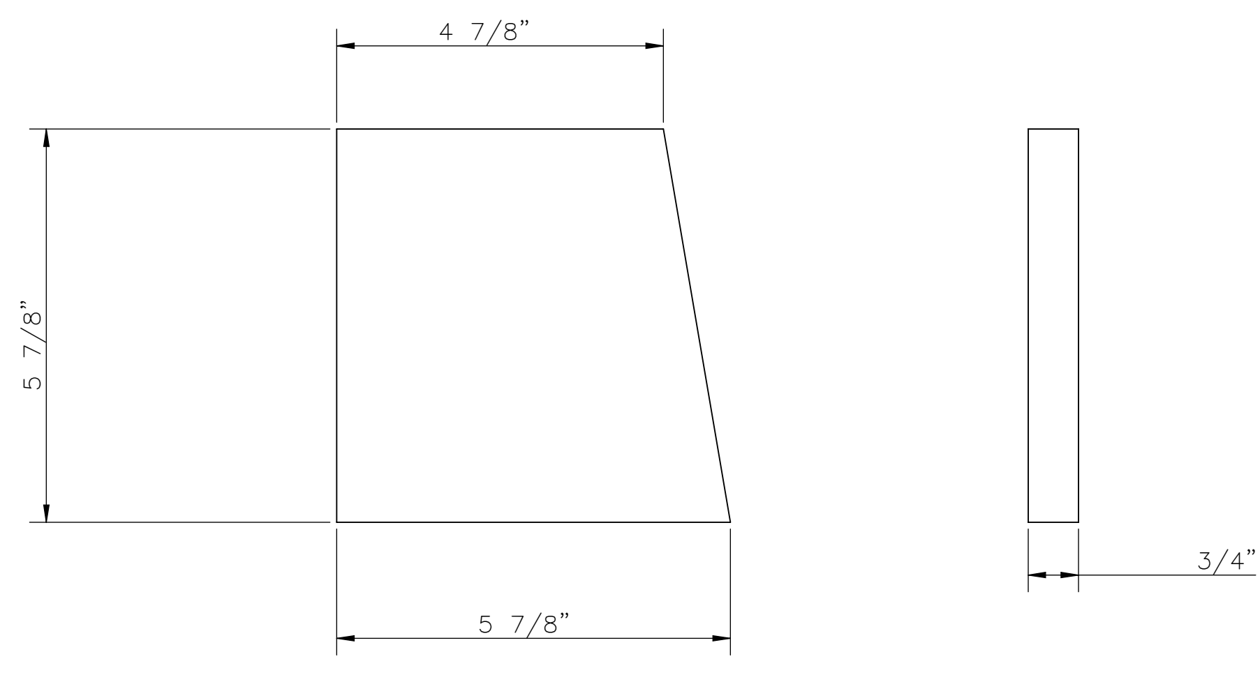
⑦ 48 INCH RISER GUSSET PLATE SCALE: 6"=1'-0"
