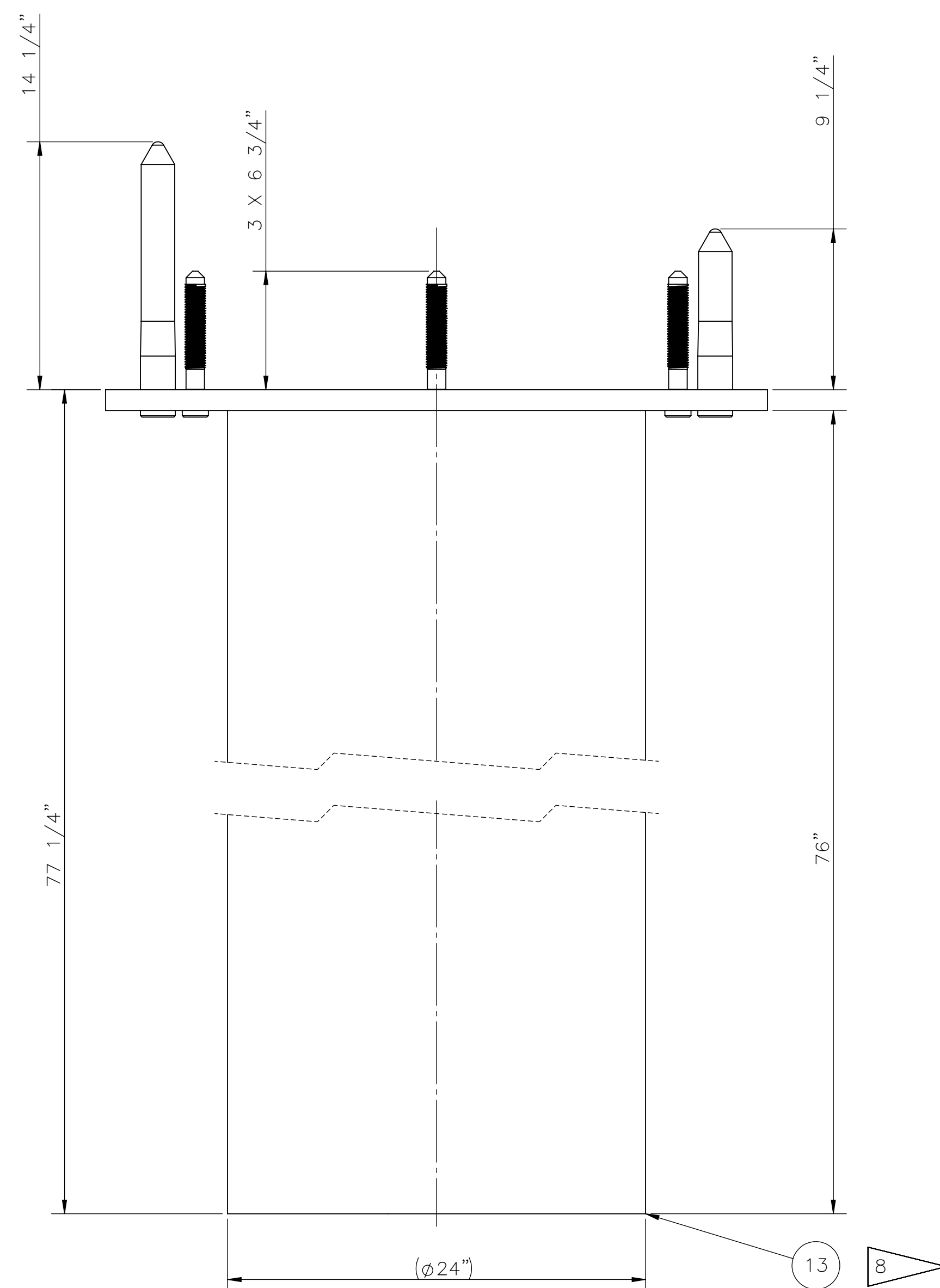
② PWST 24 INCH RISER ASSEMBLY SCALE: 2"=1'-0"
