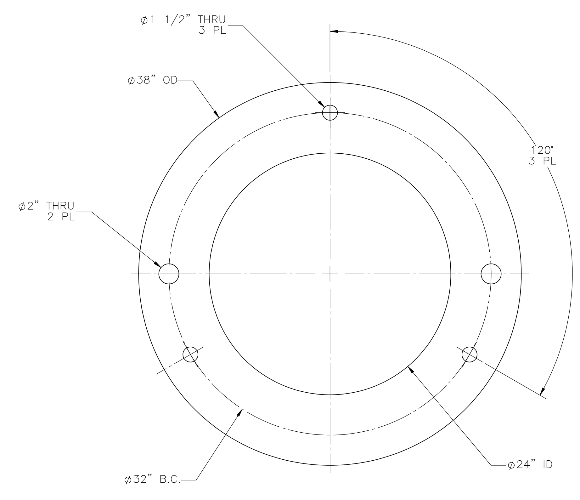
⑫ 24 INCH RISER PLATE SCALE: 2"=1'-0"
